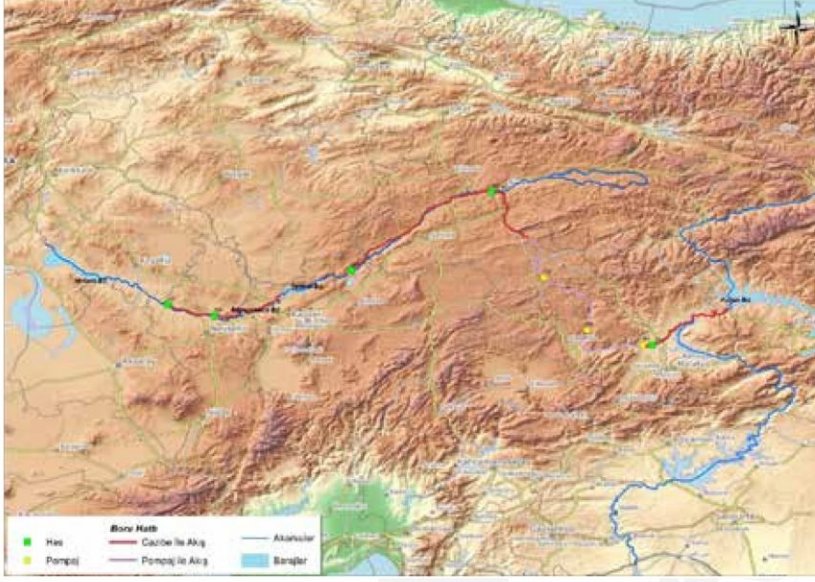
Keban Barajı – Yamula Barajı – Hirfanlı Barajı su boru hattı güzergâhı
